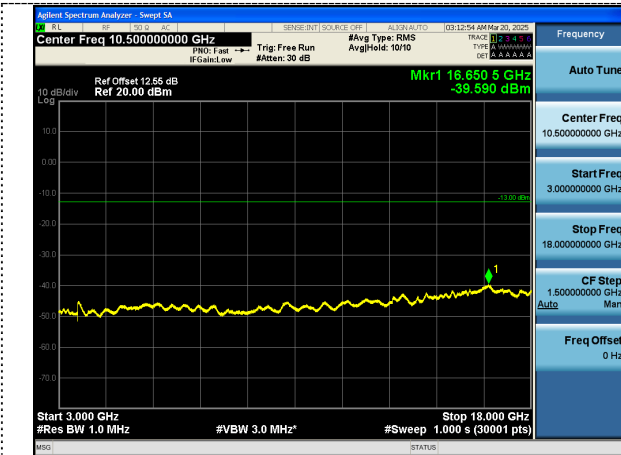
3GHz ~18GHz
