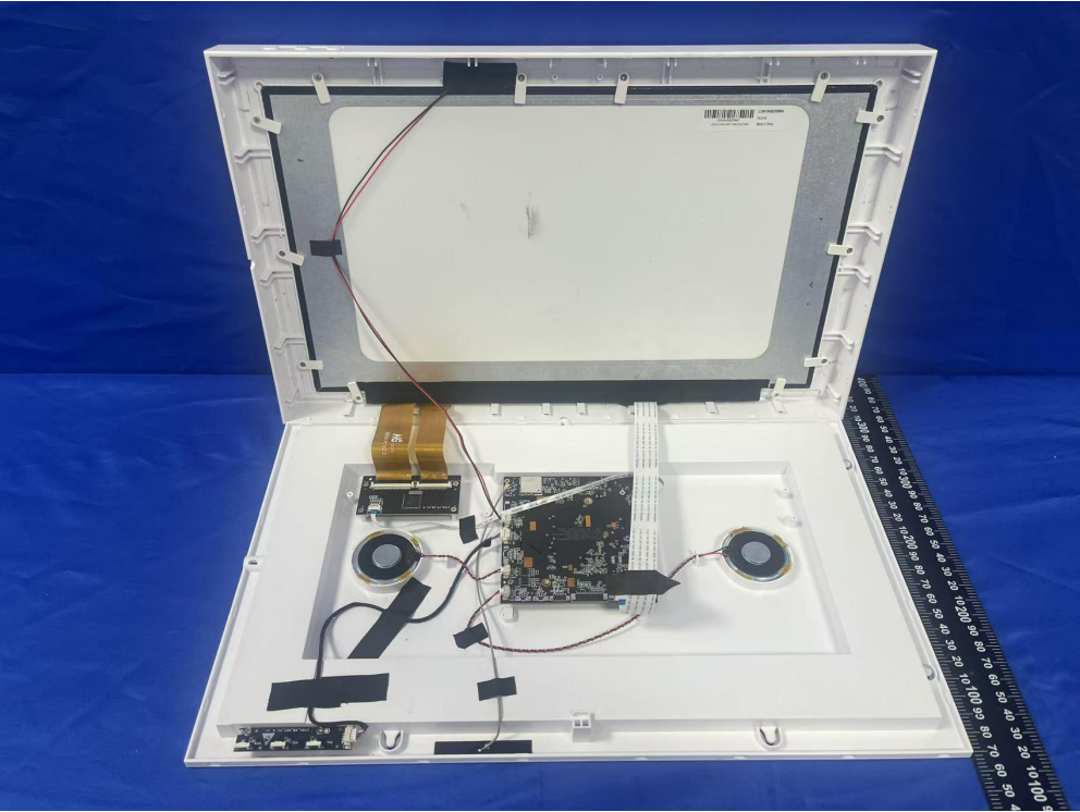
Antenna
