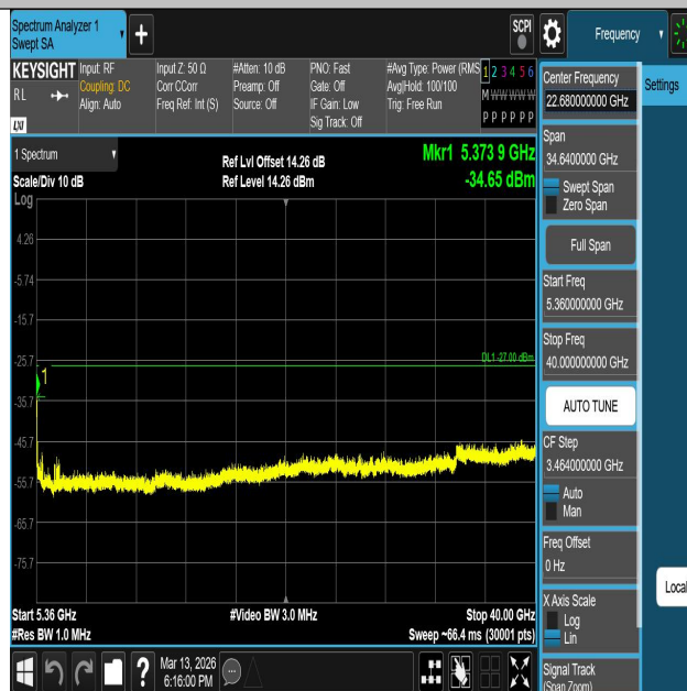
11AC80SISO-Ant1-5290-5360~40000-PASS
