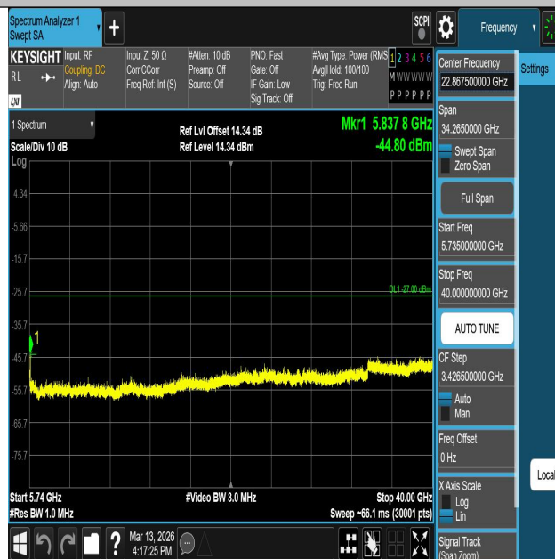
11AC20SISO-Ant1-5700-5735~40000-PASS
