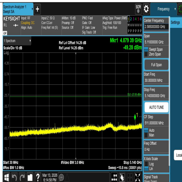
11AC80SISO-Ant1-5290-30~5140-PASS
