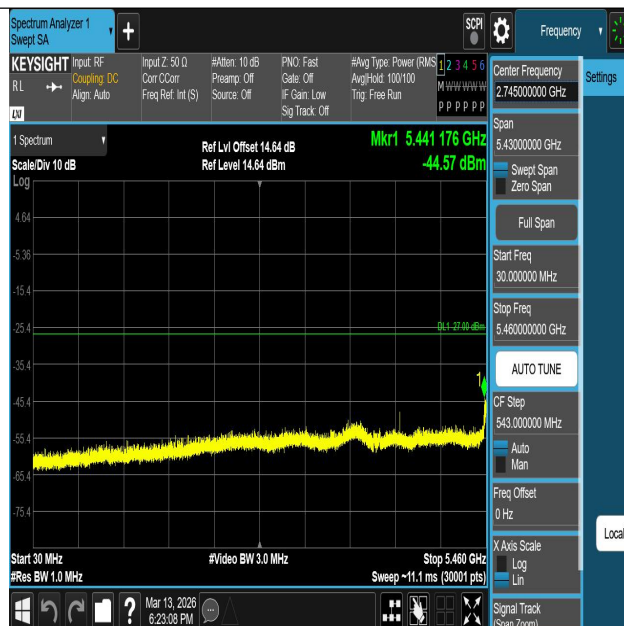
11AC80SISO-Ant1-5530-30~5460-PASS
