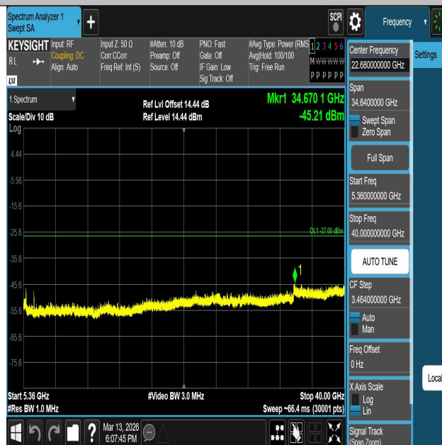
11AC80SISO-Ant1-5210-5360~40000-PASS
