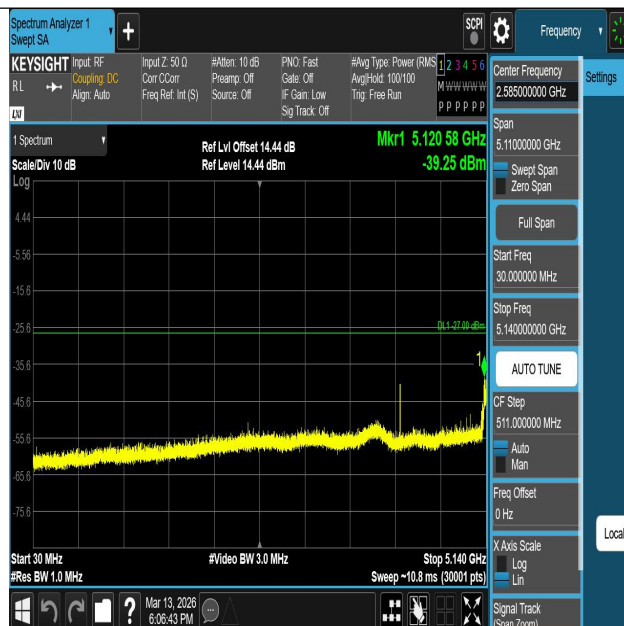
11AC80SISO-Ant1-5210-30~5140-PASS
