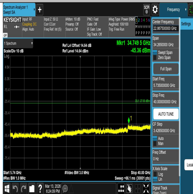
11AC80SISO-Ant1-5530-5735~40000-PASS
