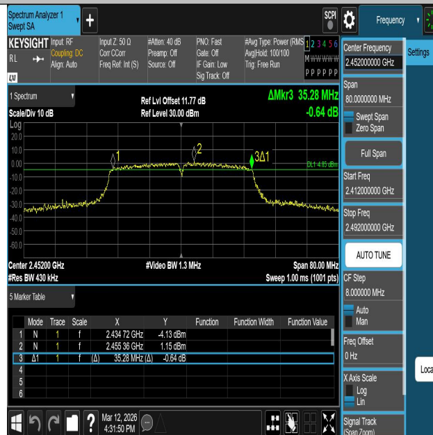
11N40ISO-Ant1-2452-PASS
