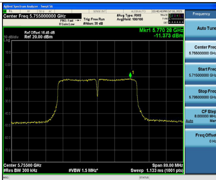
11N40ISO-Ant1-5755-PASS
