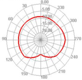
2450.000MHz H
