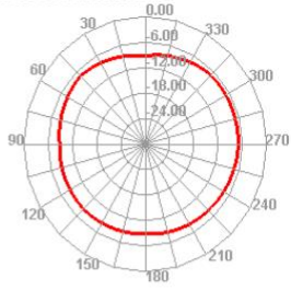
2400.000MHz E2
