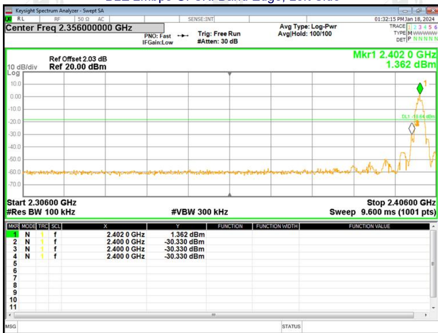
BLE 2Mbps GFSK: Band Edge, Left Side
