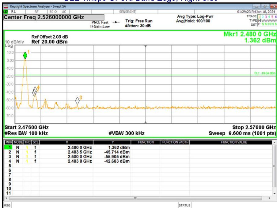
BLE 1Mbps GFSK: Band Edge, Right Side
