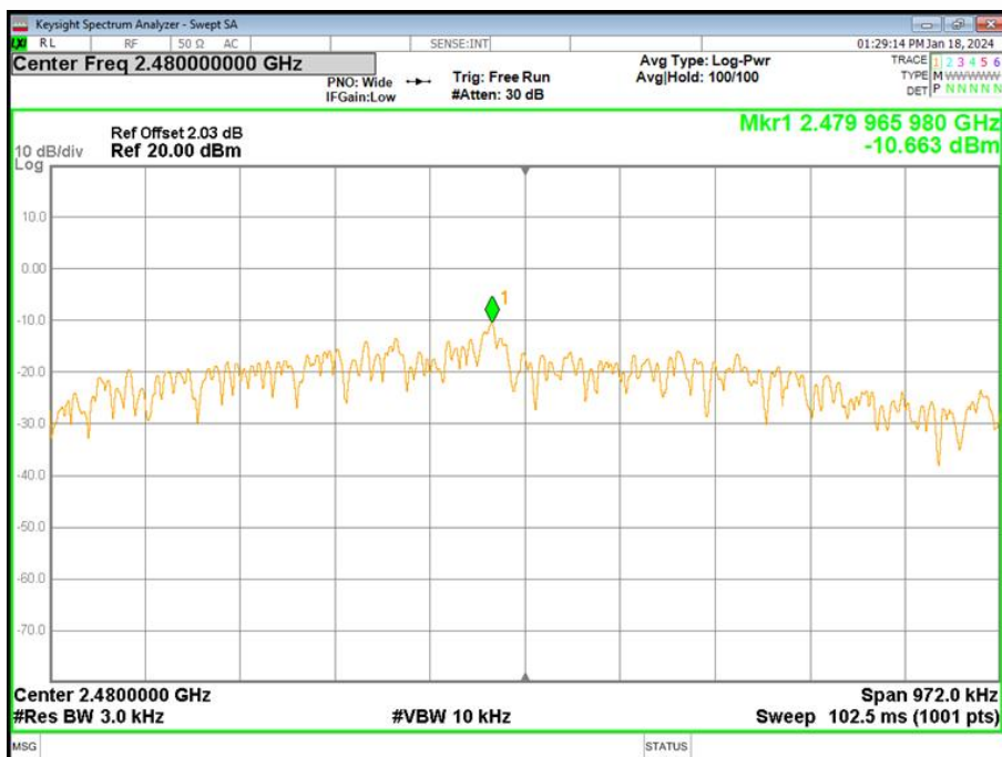
BLE 2Mbps CH40
