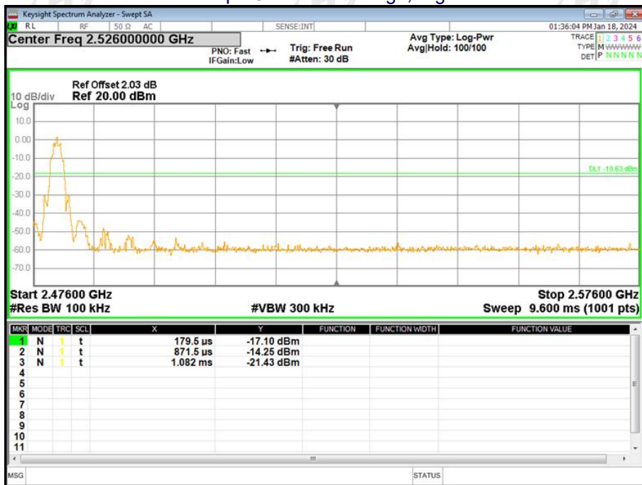
BLE 2Mbps GFSK: Band Edge, Right Side
