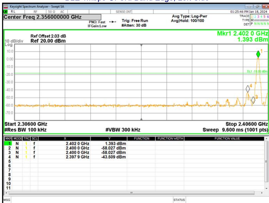
BLE 1Mbps GFSK: Band Edge, Left Side
