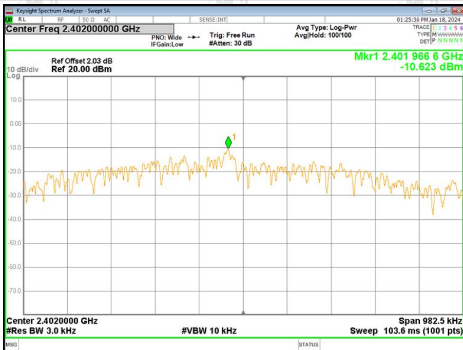
BLE 1Mbps CH01
