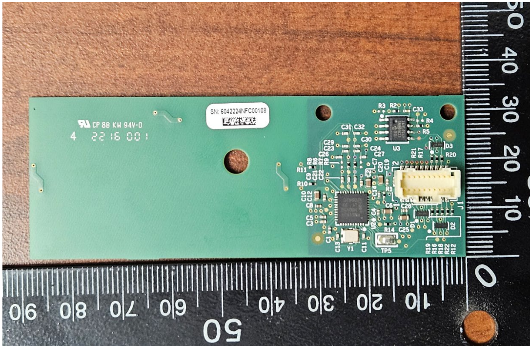
NFC Radio
