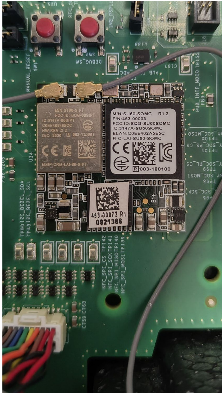
WiFi Module
