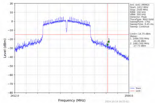
802.11n(HT40)_HCH_2452MHz_Ant1 (MIMO)_NTNV
