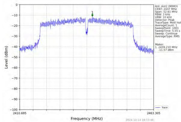
802.11n(HT40)_MCH_2437MHz_MIMO_NTNV
