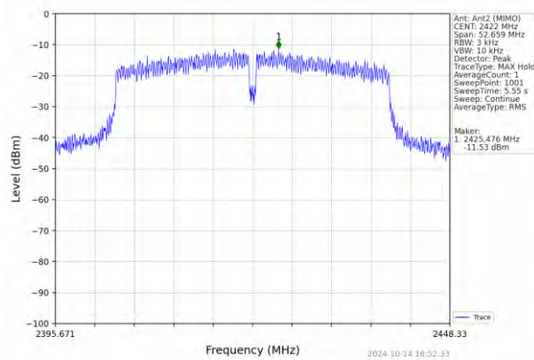
802.11n(HT40)_LCH_2422MHz_MIMO_NTNV
