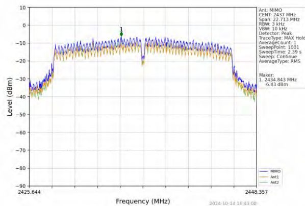
802.11n(HT20)_MCH_2437MHz_MIMO_NTNV
