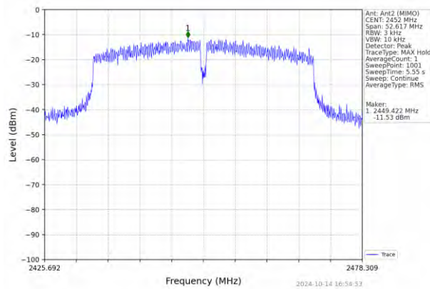
802.11n(HT40)_HCH_2452MHz_MIMO_NTNV
