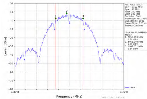
802.11b_HCH_2462MHz_Ant1 (SISO)_NTNV
