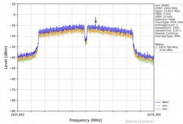
802.11n(HT40)_HCH_2452MHz_MIMO_NTNV
