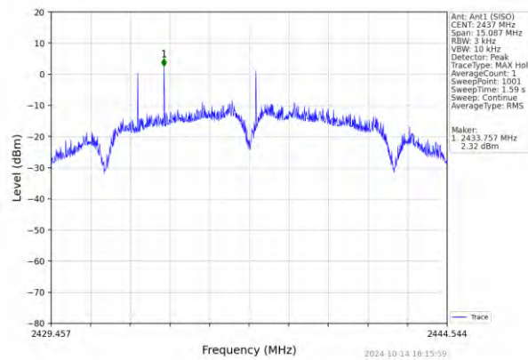
802.11b_MCH_2437MHz_Ant1 (SISO)_NTNV
