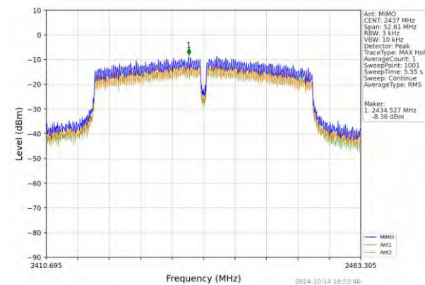
802.11n(HT40)_MCH_2437MHz_MIMO_NTNV
