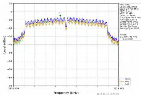
802.11n(HT20)_HCH_2462MHz_MIMO_NTNV
