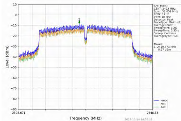
802.11n(HT40)_LCH_2422MHz_MIMO_NTNV
