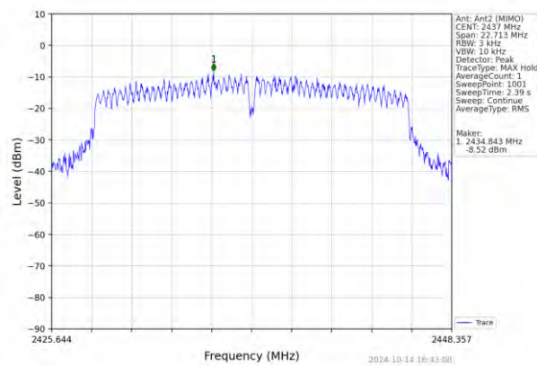
802.11n(HT20)_MCH_2437MHz_MIMO_NTNV
