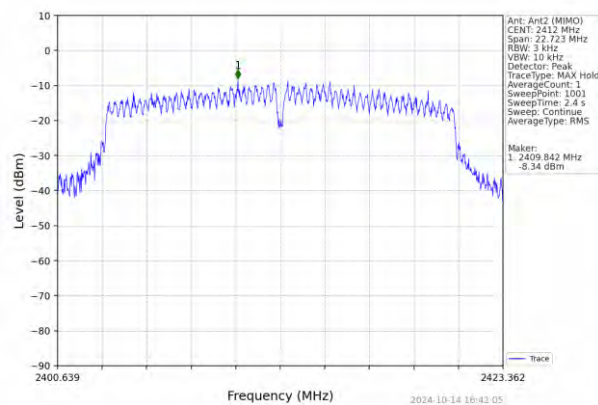
802.11n(HT20)_LCH_2412MHz_MIMO_NTNV
