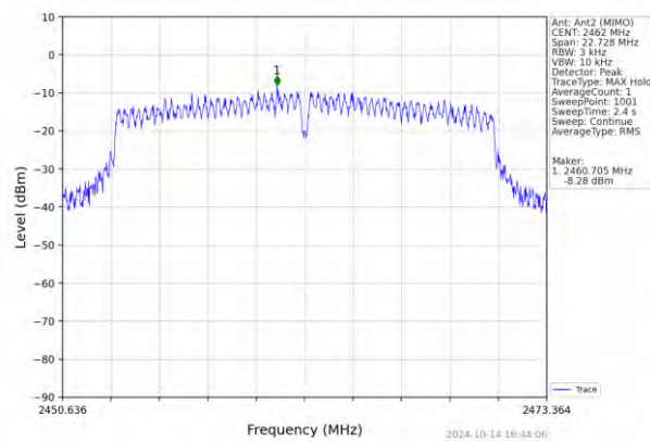
802.11n(HT20)_HCH_2462MHz_MIMO_NTNV
