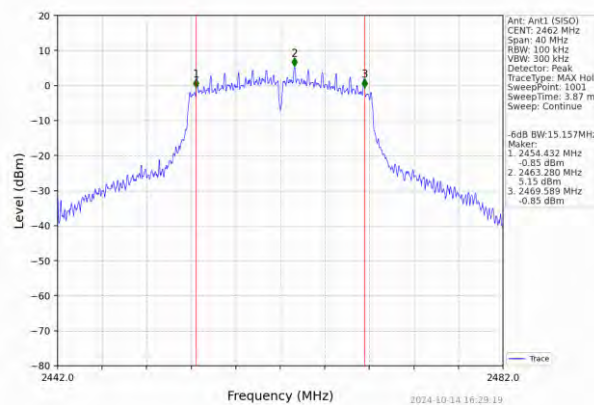
802.11g_HCH_2462MHz_Ant1 (SISO)_NTNV
