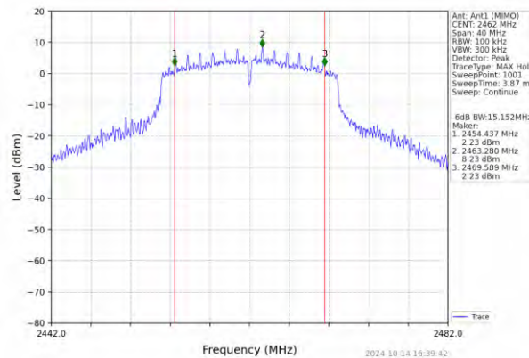
802.11n(HT20)_HCH_2462MHz_Ant1 (MIMO)_NTNV
