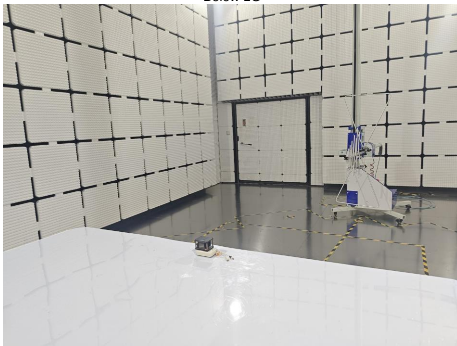
9kHz-30MHz
