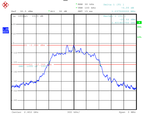
3DH1_Low 1.238MHz
