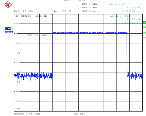
2DH5_Hopping 2.925ms
