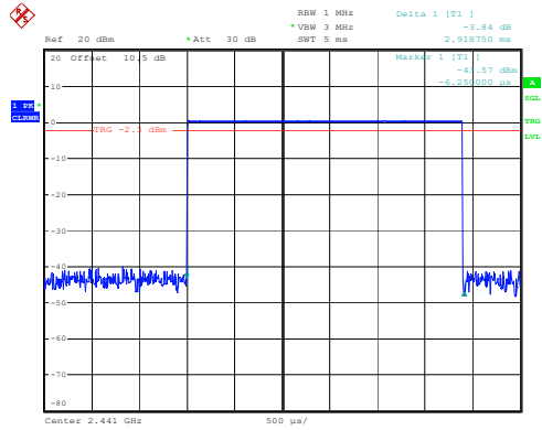
DH5_Hopping 2.919ms
