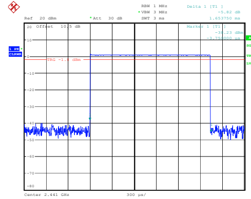
DH3_Hopping 1.654ms
