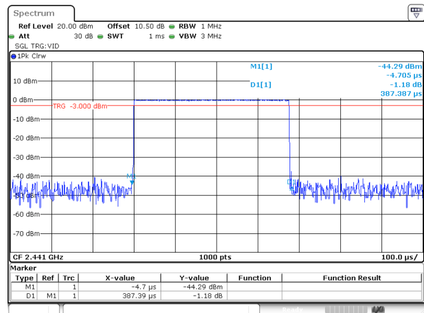
DH1_Hopping
