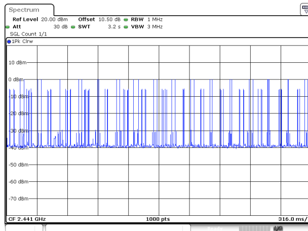
DH1_Hopping
