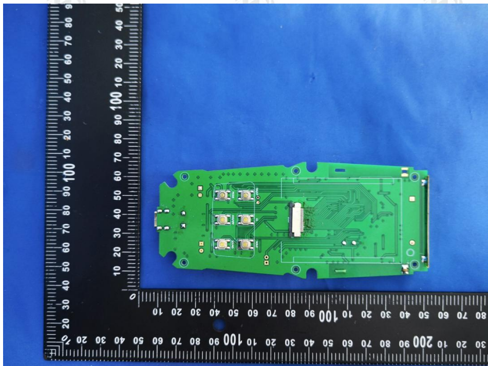
EUT Photo 10
