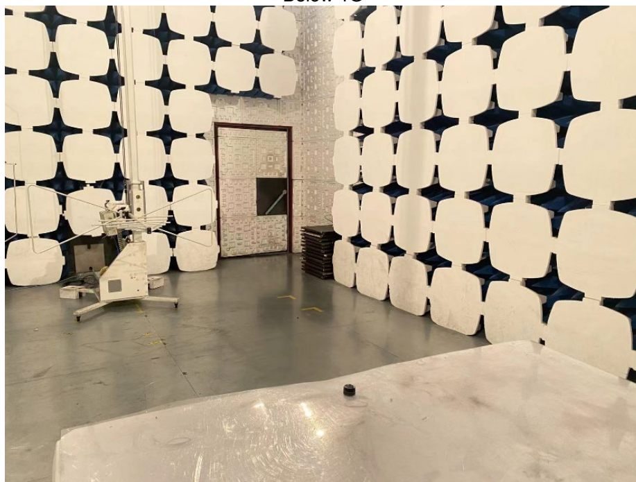
Below 1G
