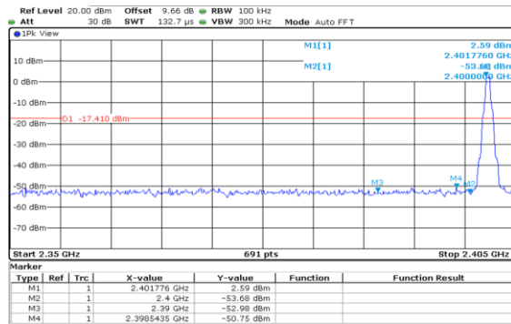
Figure 4: Band Edge
