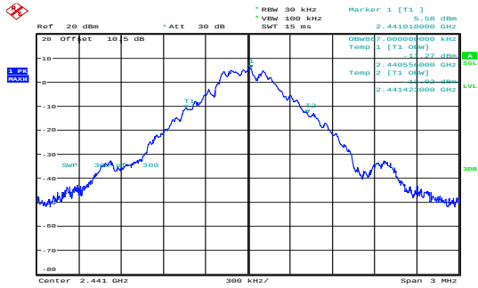
GFSK_Middle 0.867MHz
