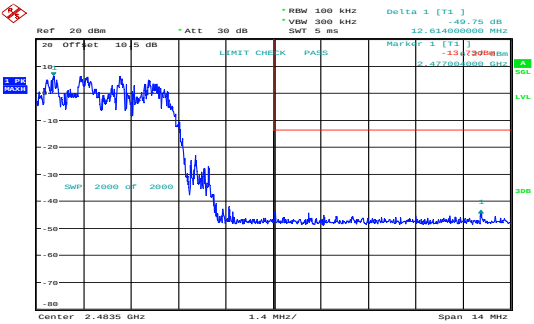
8DPSK_Hopping_Upper 49.75dB
