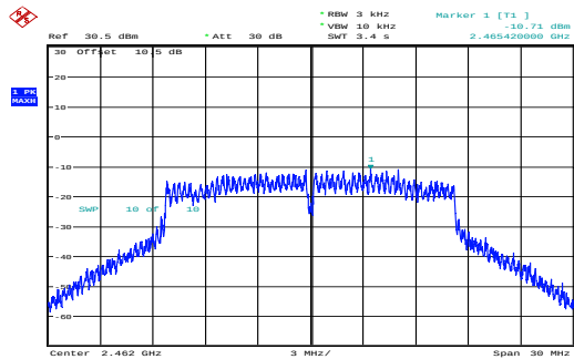
g_2462MHz_Chain 0 -10.71dBm/3kHz
