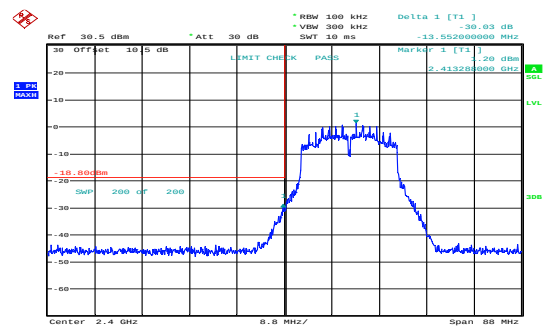
n20_2412MHz_Chain 1 30.03dB
