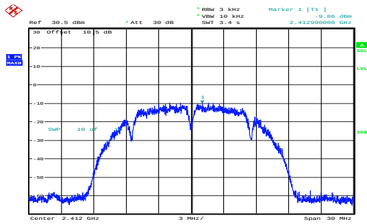
b_2412MHz_Chain 0 -9.86dBm/3kHz
