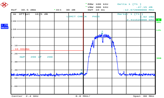
b_2412MHz_Chain 1 47.15dB
