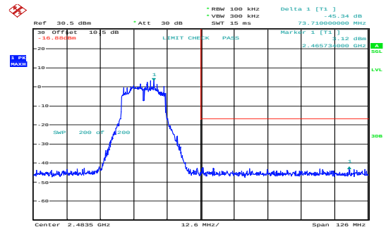
g_2462MHz_Chain 1 45.34dB
