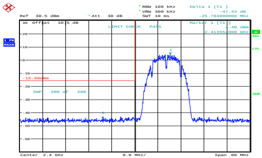
b_2412MHz_Chain 0 47.43dB
