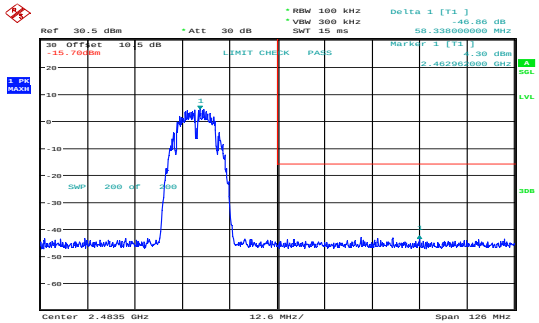
b_2462MHz_Chain 0 46.86dB
