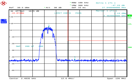
b_2462MHz_Chain 1 47.23dB
