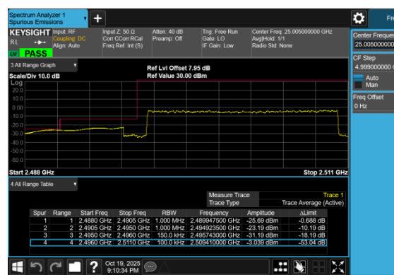
Band41_15MHz_QPSK_39725_75RB#0
