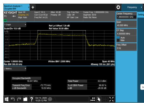
Band2-20MHz-QPSK-18900-100RB#0-PASS
