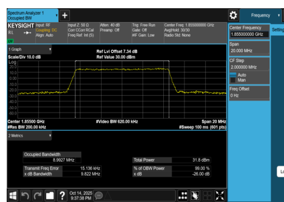
Band2-10MHz-QPSK-18650-50RB#0-PASS
