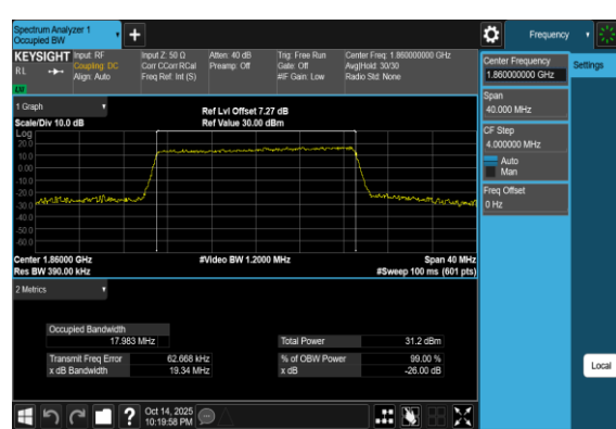
Band2-20MHz-16QAM-18700-100RB#0-PASS
