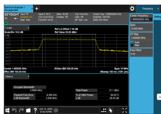
Band2-5MHz-QPSK-18900-25RB#0-PASS
