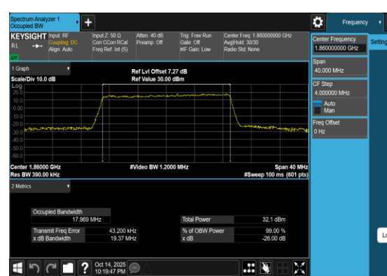
Band2-20MHz-QPSK-18700-100RB#0-PASS
