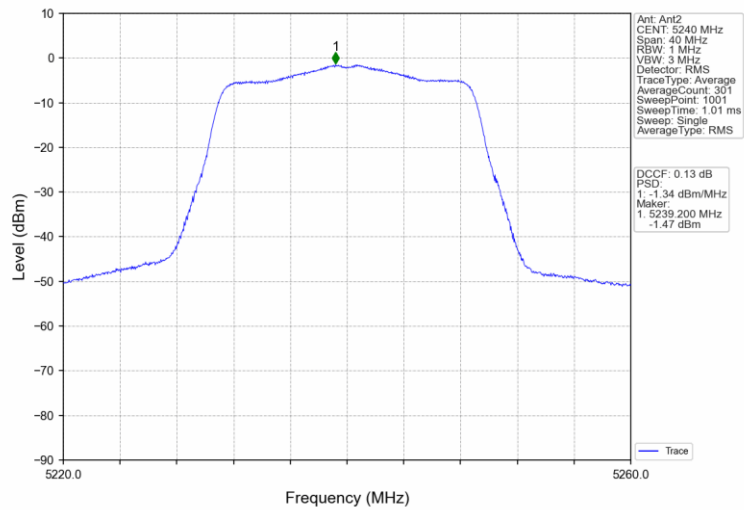
802.11n(HT20)_HCH_5240MHz_MIMO_NTNV
