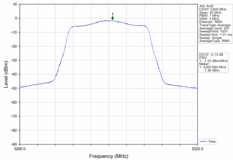
802.11n(HT20)_MCH_5300MHz_MIMO_NTNV
