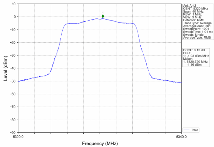
802.11n(HT20)_HCH_5320MHz_MIMO_NTNV
