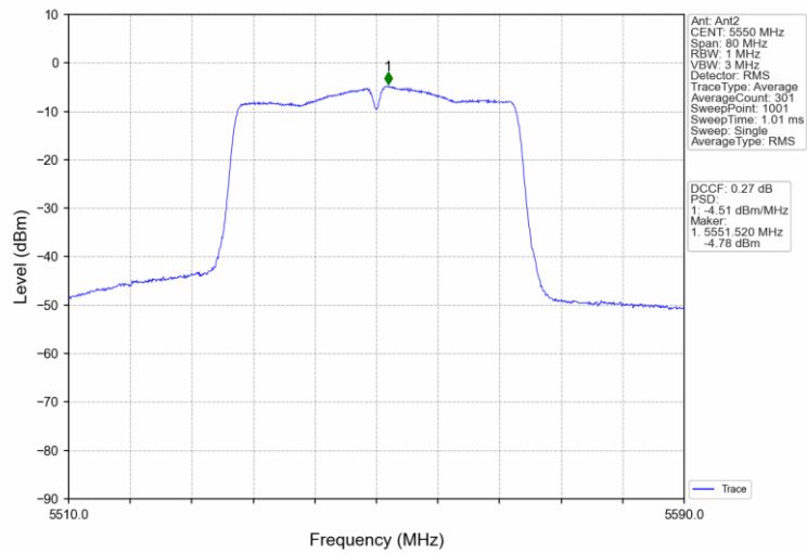
802.11n(HT40)_MCH_5550MHz_MIMO_NTNV
