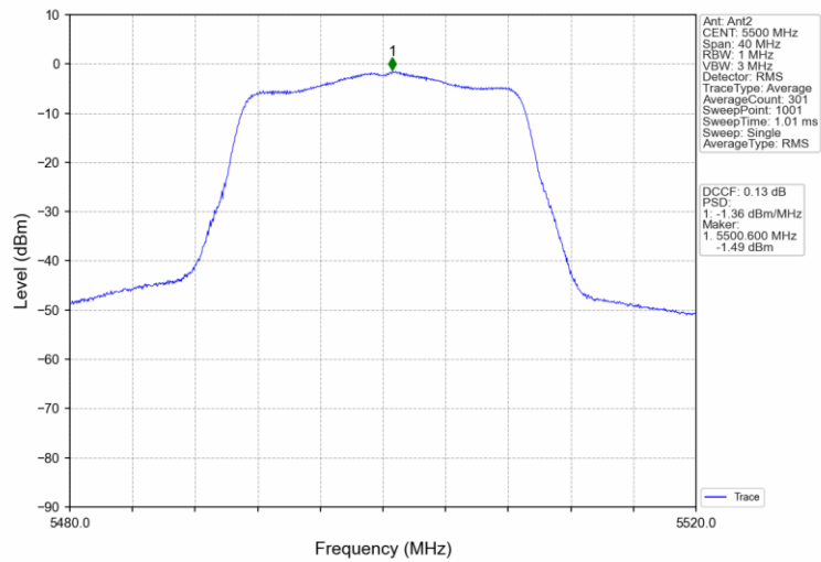
802.11n(HT20) LCH_5500MHz_MIMO_NTNV
