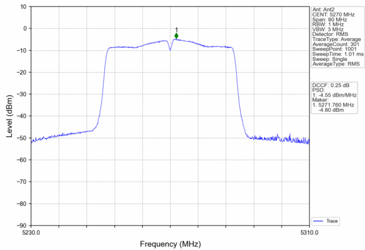
802.11n(HT40) LCH_5270MHz_MIMO_NTNV
