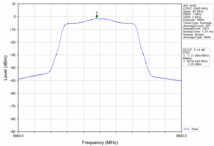
802.11n(HT20)_MCH_5580MHz_MIMO_NTNV
