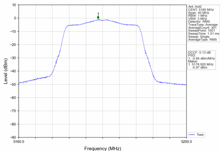
802.11n(HT20)_LCH_5180MHz_MIMO_NTNV
