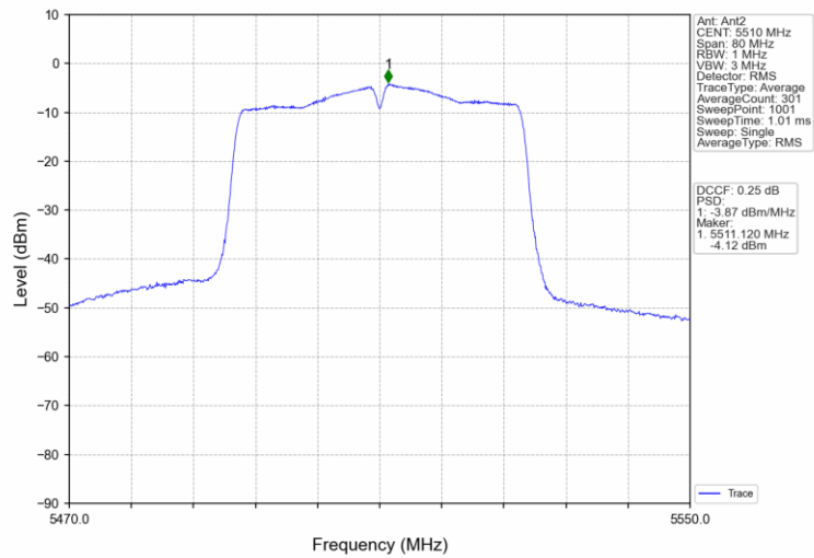
802.11n(HT40) LCH_5510MHz_MIMO_NTNV
