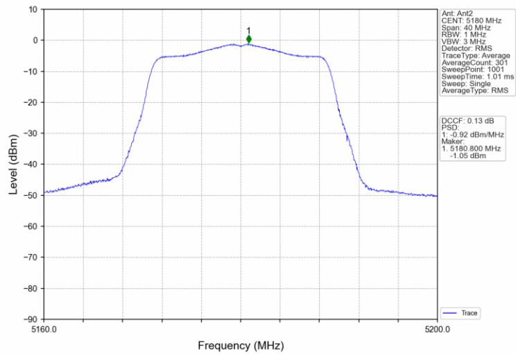
802.11ac(VHT20) LCH 5180MHz MIMO NTNv
