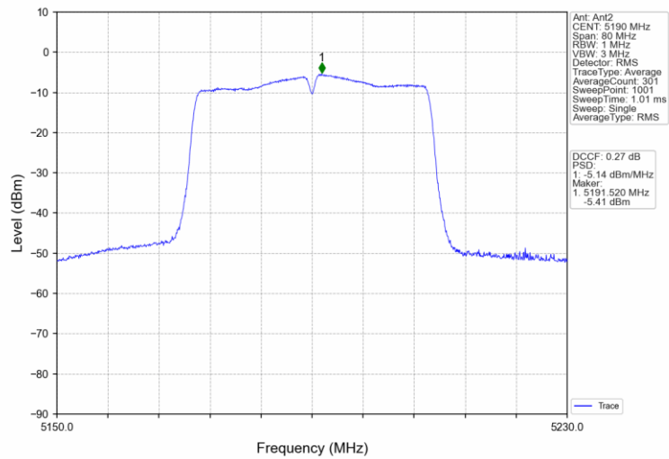
802.11n(HT40) LCH 5190MHz MIMO NTNv
