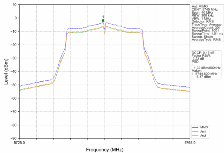
802.11n(HT20)_MCH_5785MHz_Ant1_NTNV
