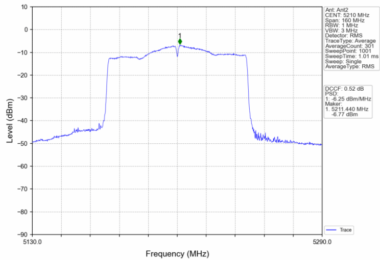
802.11ac(VHT80)_MCH_5210MHz_MIMO_NTNV
