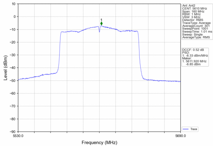
802.11ac(VHT80)_HCH_5610MHz_MIMO_NTNV
