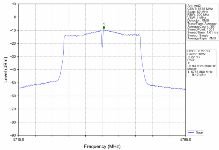
802.11n(HT40)_LCH_5755MHz_MIMO_NTNV
