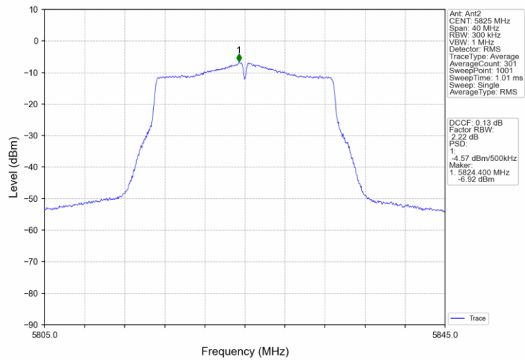
802.11n(HT20)_HCH_5825MHz_MIMO_NTNV
