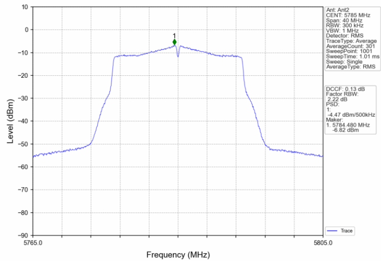
802.11n(HT20)_MCH_5785MHz_MIMO_NTNV
