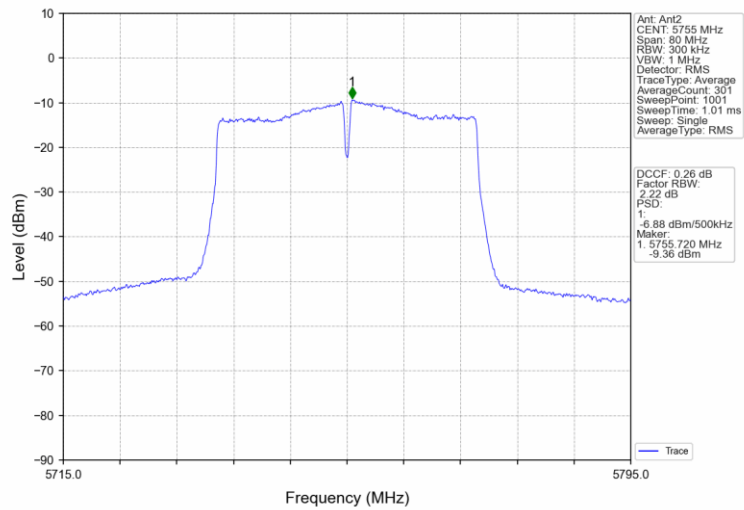
802.11ac(VHT40)_LCH_5755MHz_MIMO_NTNV
