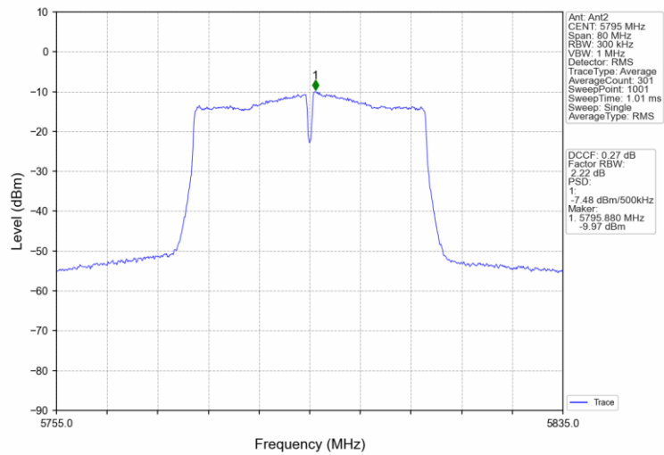
802.11n(HT40)_HCH_5795MHz_MIMO_NTNV
