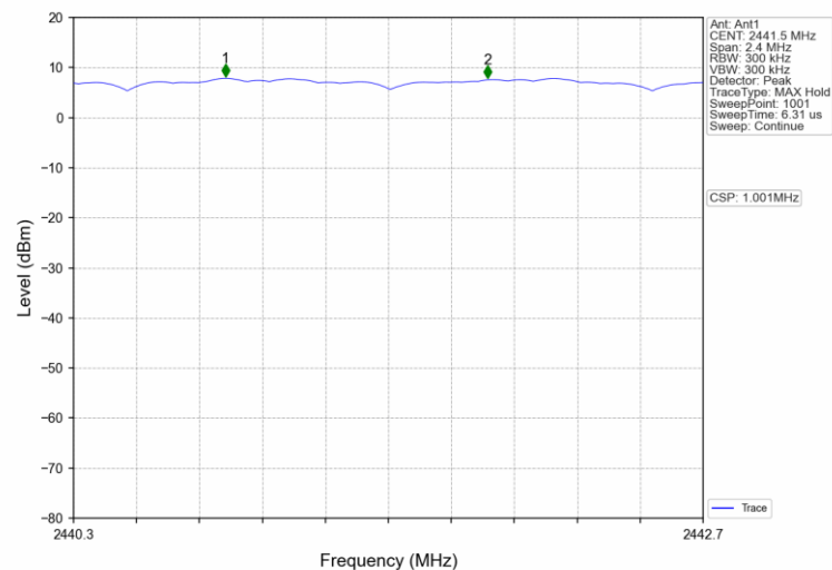
Pi/4DQPSK_2DH5_HOPP_Ant1_NTNV
