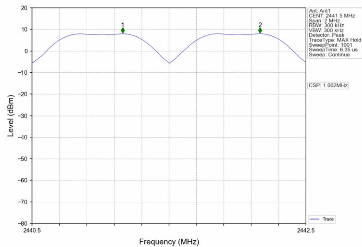
Pi/4DQPSK_2DH5_HOPP_Ant1_NTNV
