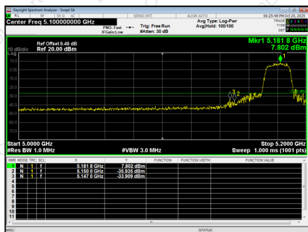
802.11ac HT20
