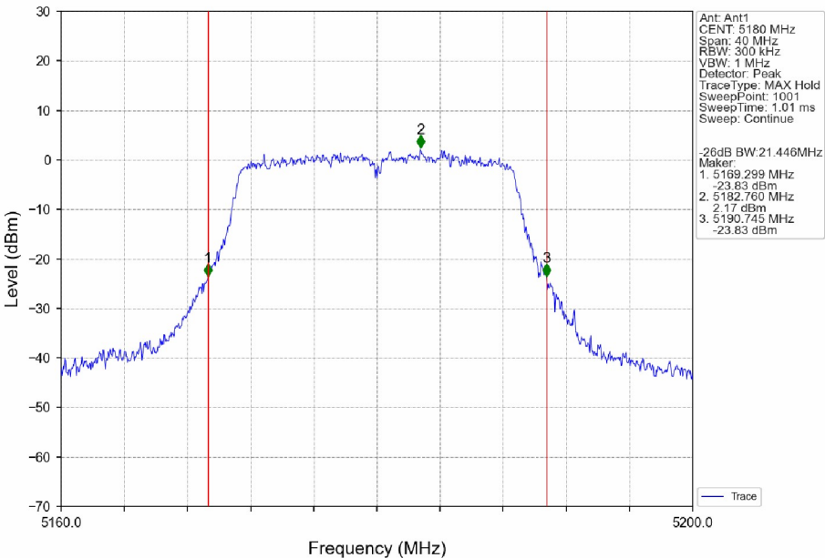
802.11n(HT20)_LCH_5180MHz_Ant1_NTNV
