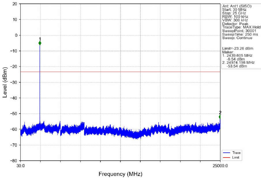
802.11n(HT20)_HCH_2462MHz_Ant1 (SISO)_NTNV
