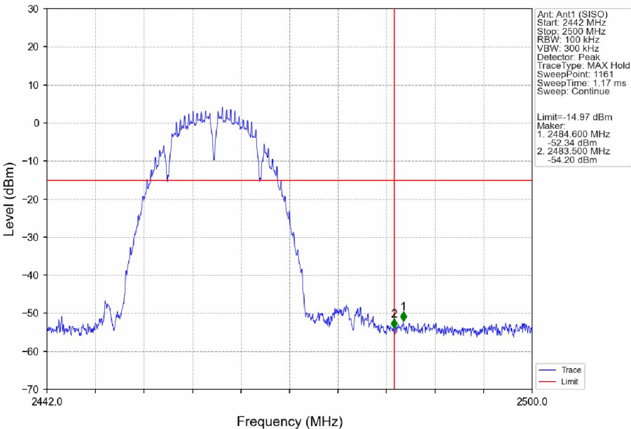
802.11b_HCH_2462MHz_Ant1 (SISO)_NTNV
