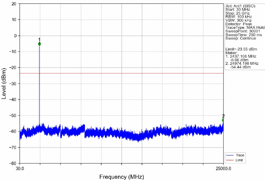
802.11g_MCH_2437MHz_Ant1 (SISO)_NTNV
