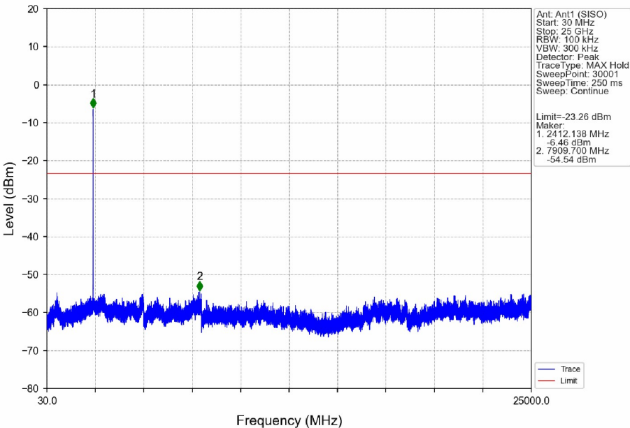
802.11n(HT20)_LCH_2412MHz_Ant1 (SISO)_NTNV
