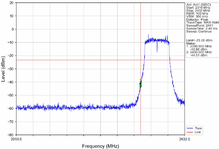
802.11n(HT20)_LCH_2412MHz_Ant1 (SISO)_NTNV
