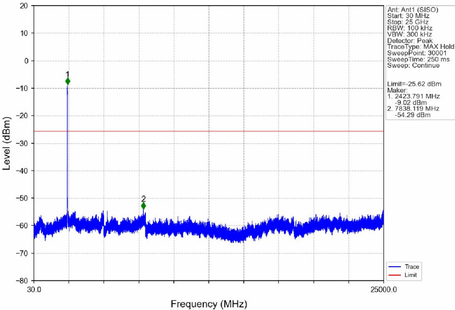
802.11n(HT40)_MCH_2437MHz_Ant1 (SISO)_NTNV
