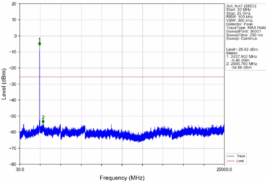
802.11n(HT40)_MCH_2437MHz_Ant1 (SISO)_NTNV
