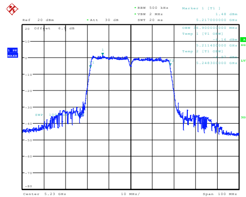
n40_5230MHz_Chain 0 36.900MHz
