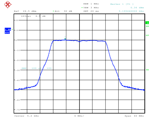
a_5200MHz_Chain 0 0.36dBm/MHz
