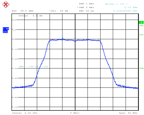
a_5240MHz_Chain 0 0.19dBm/MHz
