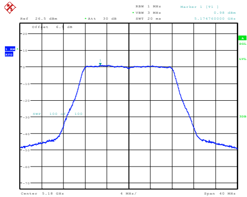
a_5180MHz_Chain 0 0.98dBm/MHz
