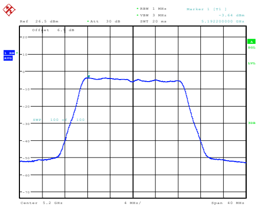
n20_5200MHz_Chain 0 -3.64dBm/MHz
