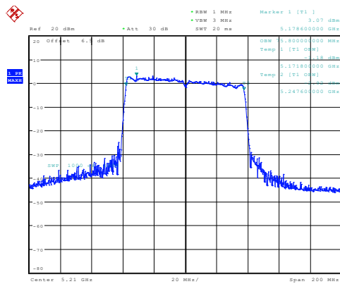
ac80_5210MHz_Chain 0 75.800MHz
