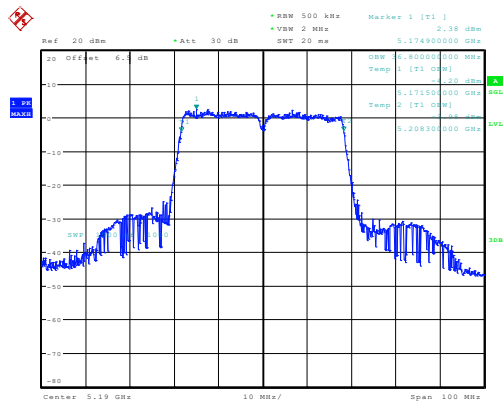
n40_5190MHz_Chain 0 36.800MHz
