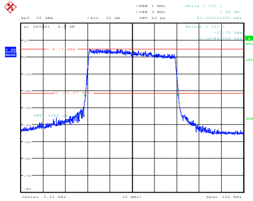
ax80_5210MHz_Chain 0 83.600MHz
