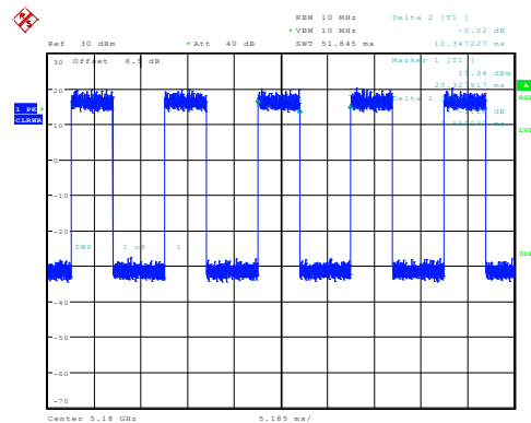
ax20_5180MHz_Chain 0 4.650ms,10.347ms
