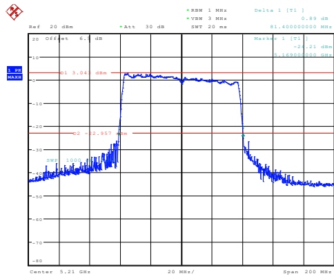
ac80_5210MHz_Chain 0 81.400MHz
