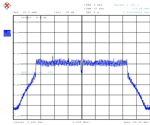
n20_2462MHz_Chain 0 -14.66dBm/3kHz
