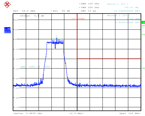
g_2462MHz_Chain 0 45.01dB
