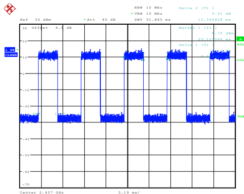
ax20_2437MHz_Chain 0 4.649ms,10.347ms
