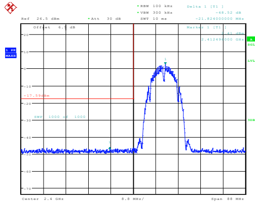
b_2412MHz_Chain 0 48.52dB
