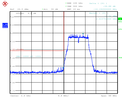
g_2412MHz_Chain 0 39.88dB
