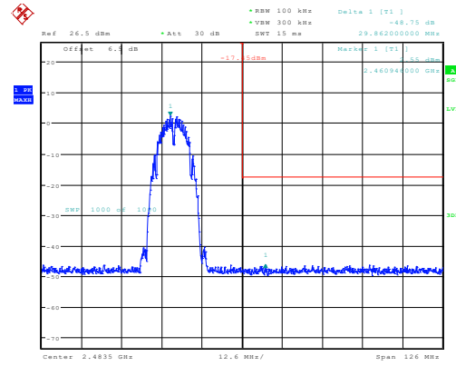
b_2462MHz_Chain 0 48.75dB
