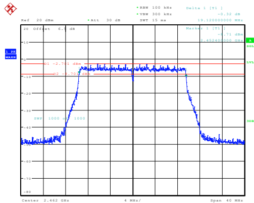
ax20_2462MHz_Chain 0 19.120MHz
