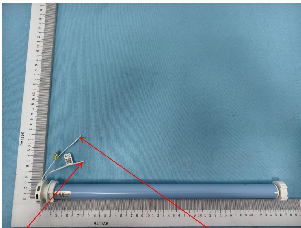
2.4G-ANT
