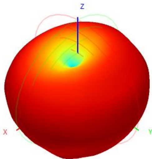
远场方向图
