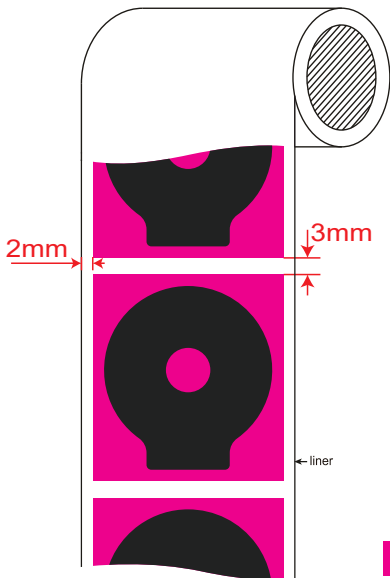
模切示意图
