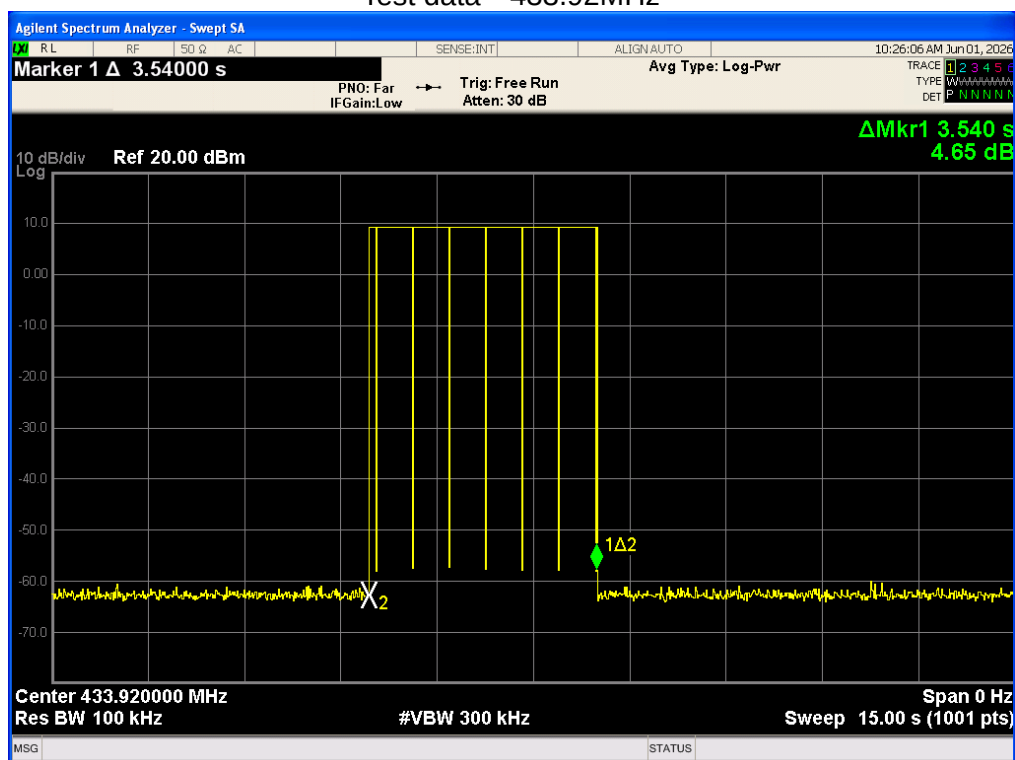
Test data—433.92MHz
