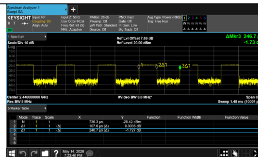
BLE 1M_Channel 19
