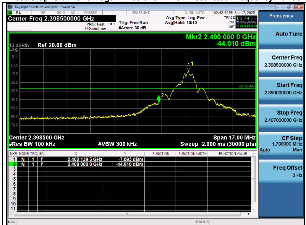
Test_Graph_GFSK_ANT1_2402_SRD_Lower Band Edge Emissions
