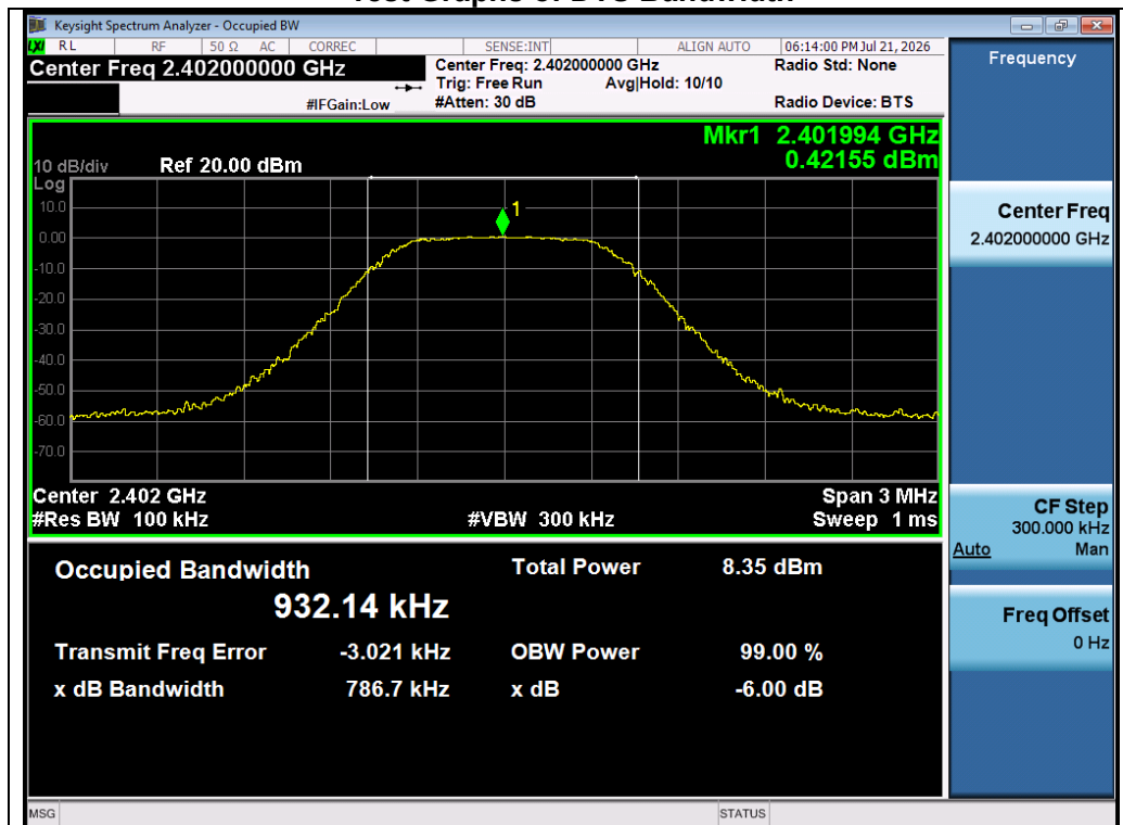
Test_Graph_2.4G_GFSK_ANT1_2402_DTSBW
