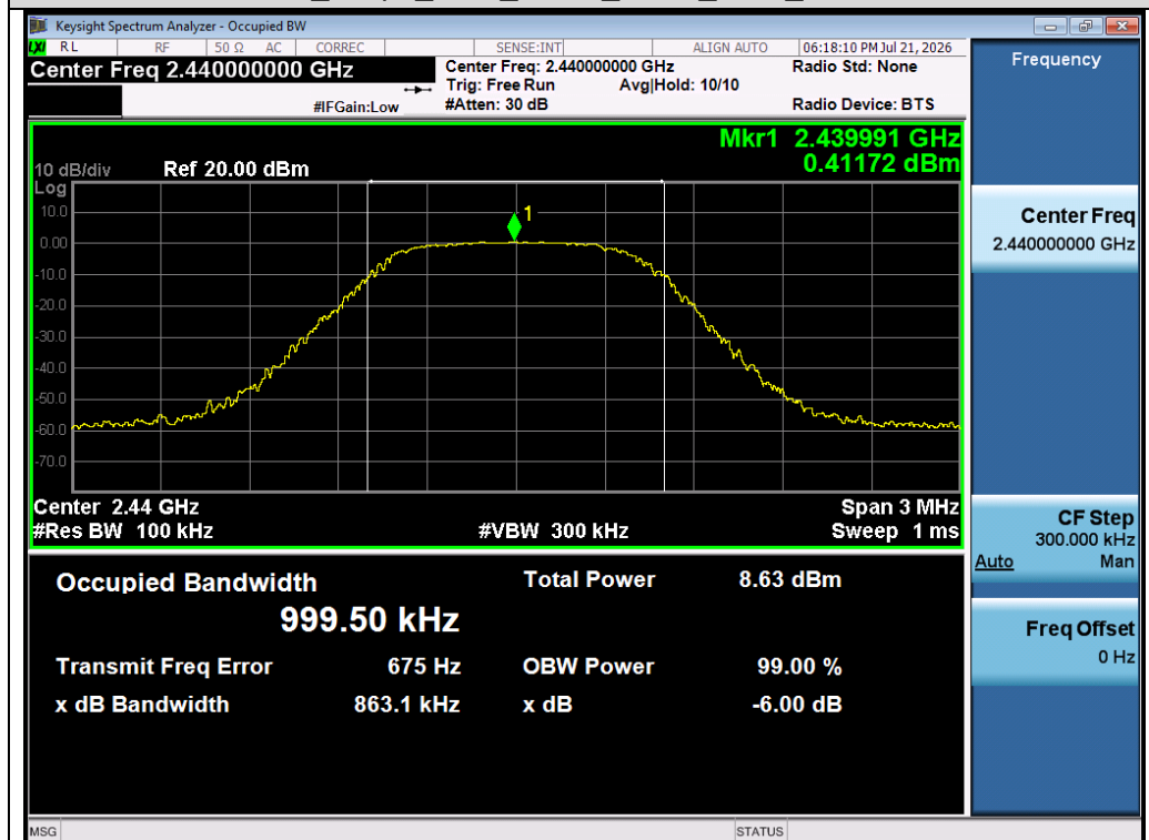
Test_Graph_2.4G_GFSK_ANT1_2440_DTSBW
