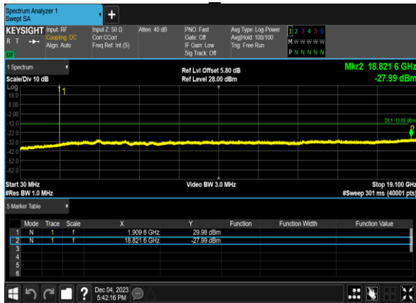
EGPRS1900 Channel810
