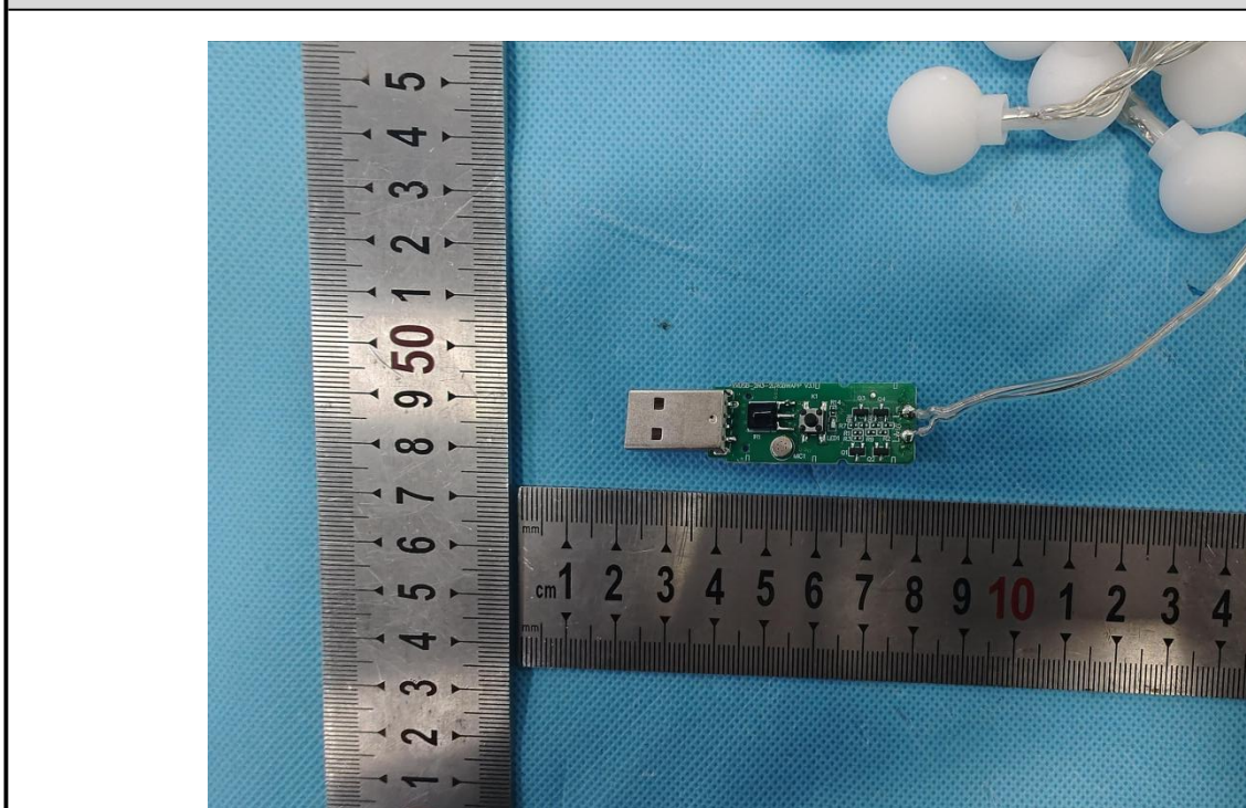
EUT Photo
