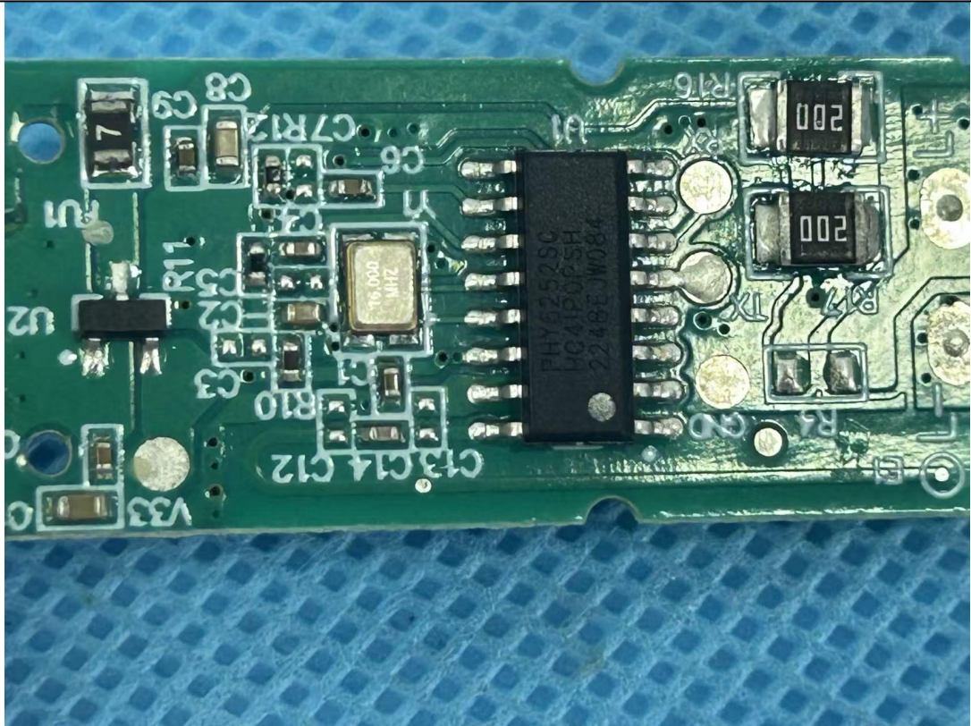
EUT Photo
