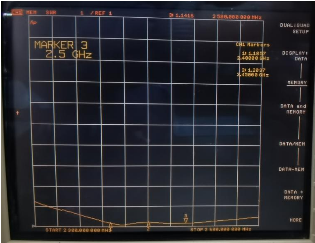
三.驻波比测试图
