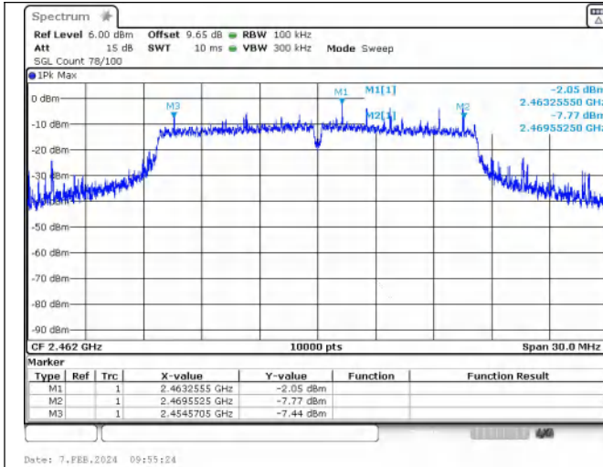
IEEE 802.11ax_Channel 11_20MHz_Antenna 0_RU&amp;Index SU
