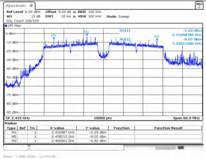
IEEE 802.11ax_Channel 3_40MHz_Antenna 0_RU&amp;Index SU
