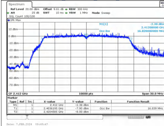
IEEE 802.11ax_Channel 1_20MHz_Antenna 0_RU&amp;Index SU
