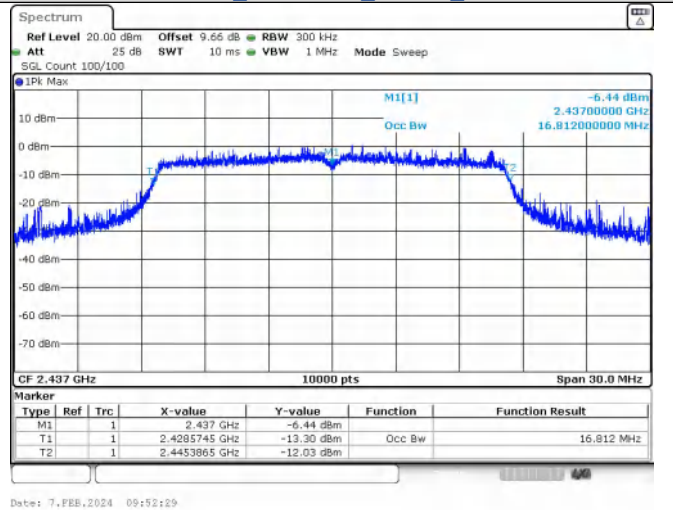
IEEE 802.11ax_Channel 6_20MHz_Antenna 0_RU&amp;Index SU
