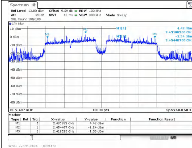
IEEE 802.11ax_Channel 6_40MHz_Antenna 0_RU&amp;Index SU
