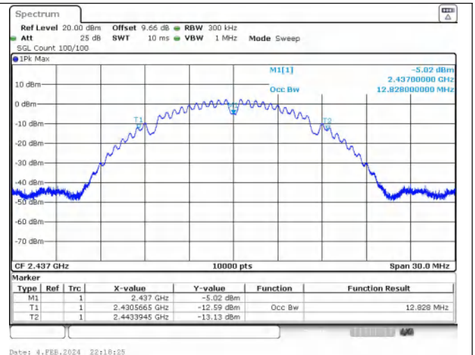
IEEE 802.11b_Channel 6_20MHz_Antenna 0
