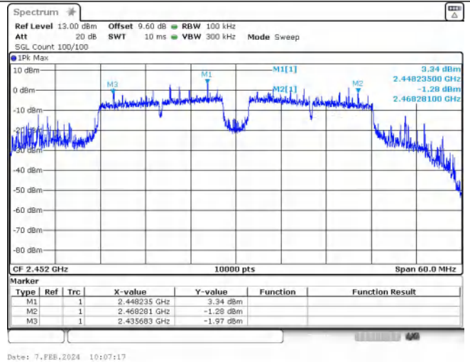
IEEE 802.11ax_Channel 9_40MHz_Antenna 0_RU&amp;Index SU
