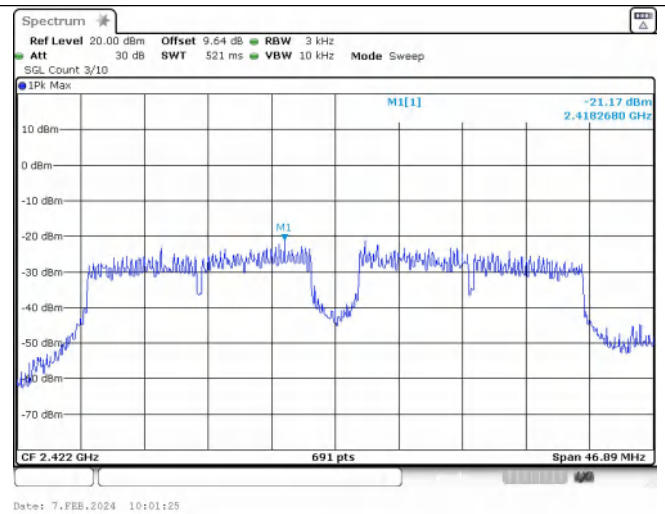
IEEE 802.11ax_Channel 3_40MHz_Antenna 0_RU&Index SU
