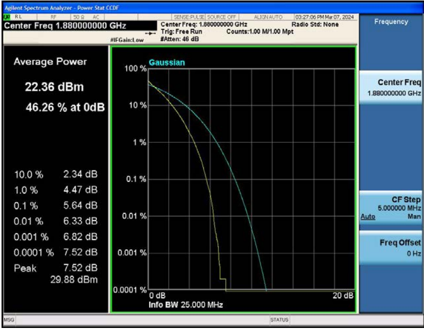
Band2-20MHz-QPSK-19100-1RB#0
