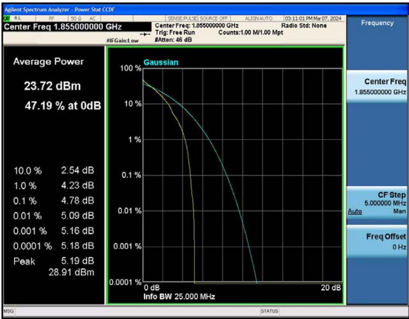
Band2-10MHz-QPSK-18650-50RB#0
