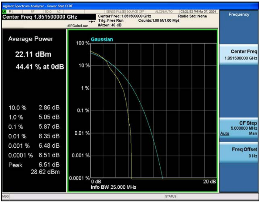
Band2-3MHz-16QAM-18615-15RB#0
