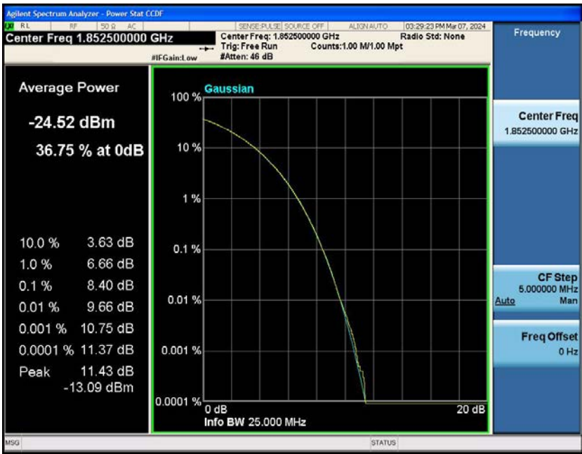
Band2-5MHz-QPSK-18625-25RB#0
