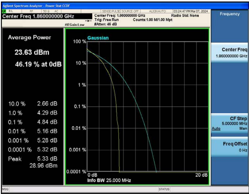
Band2-20MHz-QPSK-18700-100RB#0
