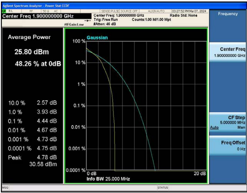
Band2-20MHz-QPSK-19100-100RB#0
