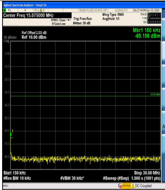
Band2-20MHz-16QAM-18900-1RB#0-1000~300 0-PASS
