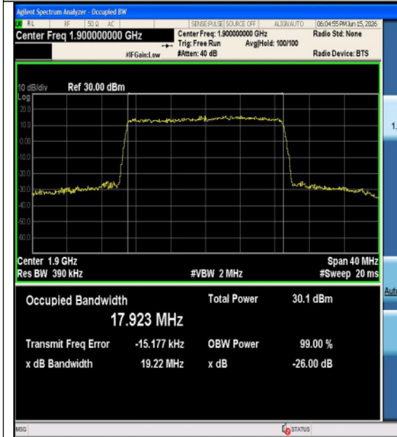
Band2-20MHz-QPSK-19100-100RB#0-PASS
