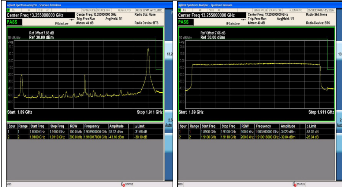
Band2-20MHz-16QAM-19100-1RB#0-PASS
