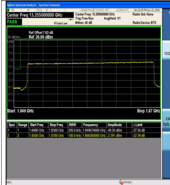
Band2-20MHz-16QAM-18700-1RB#99-PASS
