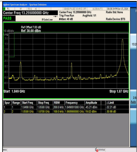
Band2-20MHz-16QAM-18700-1RB#0-PASS
