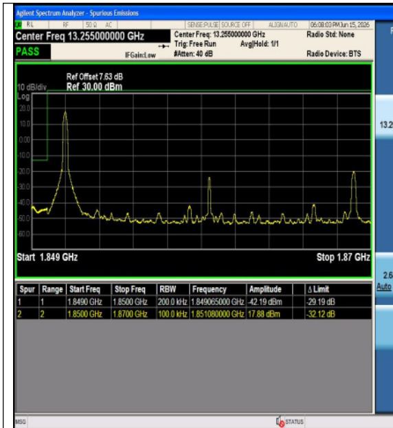
Band2-20MHz-QPSK-18700-100RB#0-PASS
