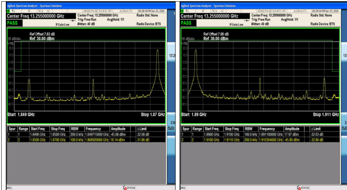
Band2-20MHz-QPSK-19100-1RB#99-PASS
