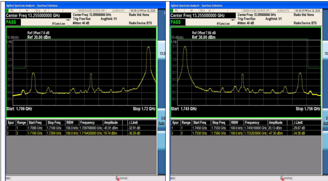
Band4-10MHz-QPSK-20350-1RB#49-PASS
