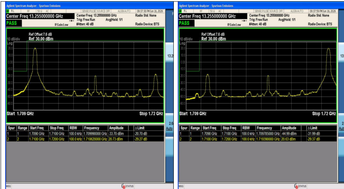
Band4-10MHz-QPSK-20000-50RB#0-PASS
