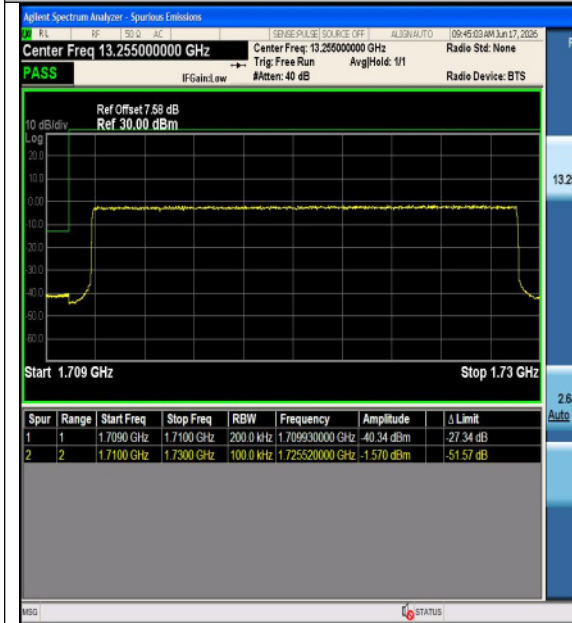
Band4-20MHz-16QAM-20050-1RB#99-PASS
