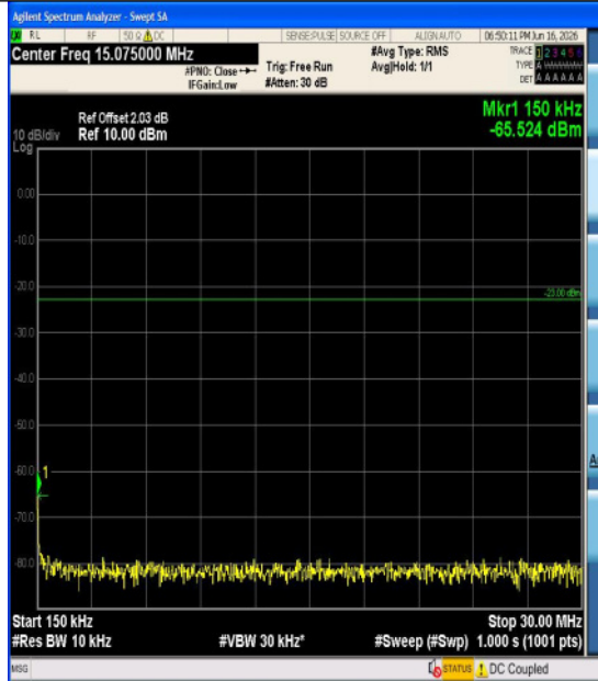
Band5-3MHz-QPSK-20635-1RB#0-1000~3000-P ASS
