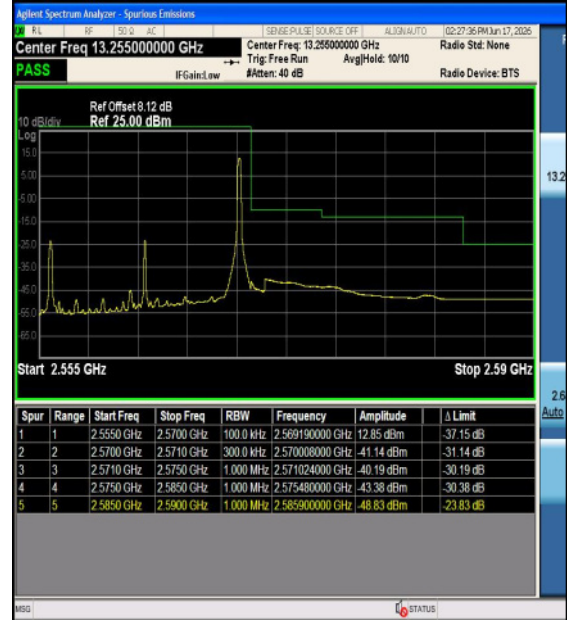
Band7-20MHz-QPSK-20850-1RB#99-PASS
