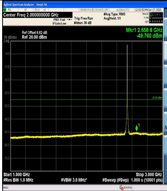
Band7-5MHz-QPSK-21100-25RB#0-18000~270
