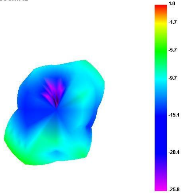
2410.000MHz E1
