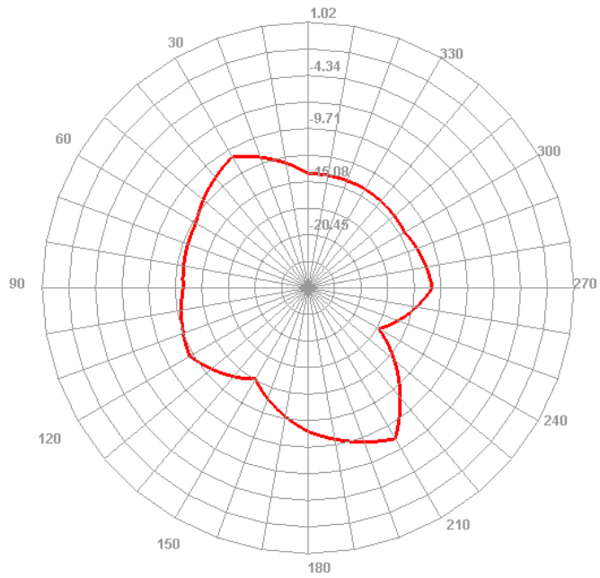
2410.000MHz E1
