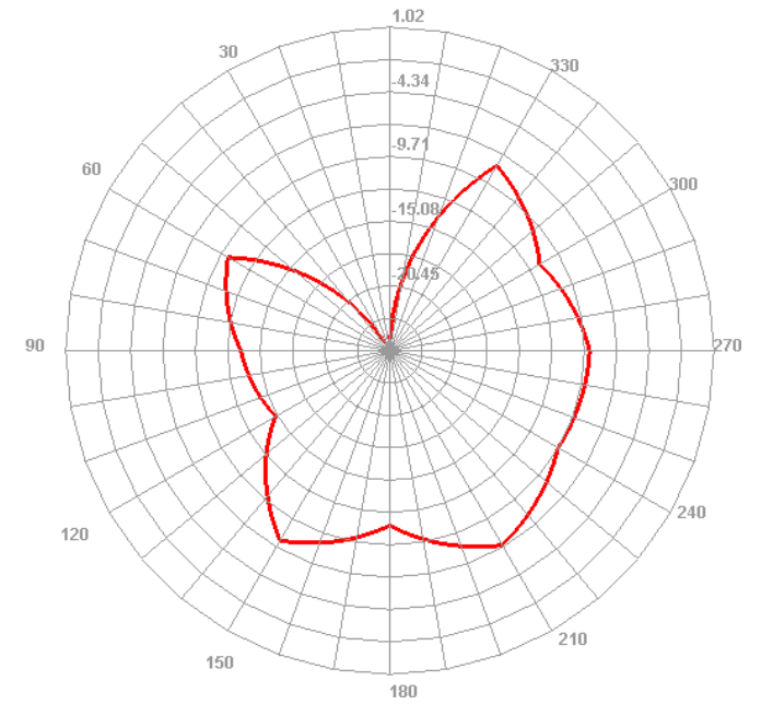
2410.000MHz E2
