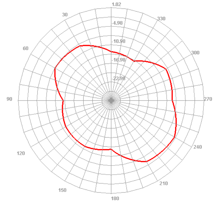
2410.000MHz H
